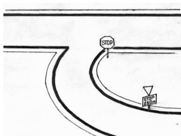
Рис. 1.70. Схема установки знака «Уступить дорогу» с табличкой 7.1.2 и знака «Движение без остановки запрещено»
