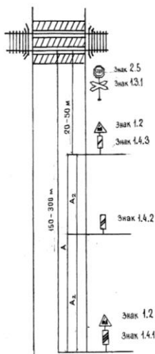
Рис. 1.2. Схема расстановки знаков у железнодорожного переезда без шлагбаума
