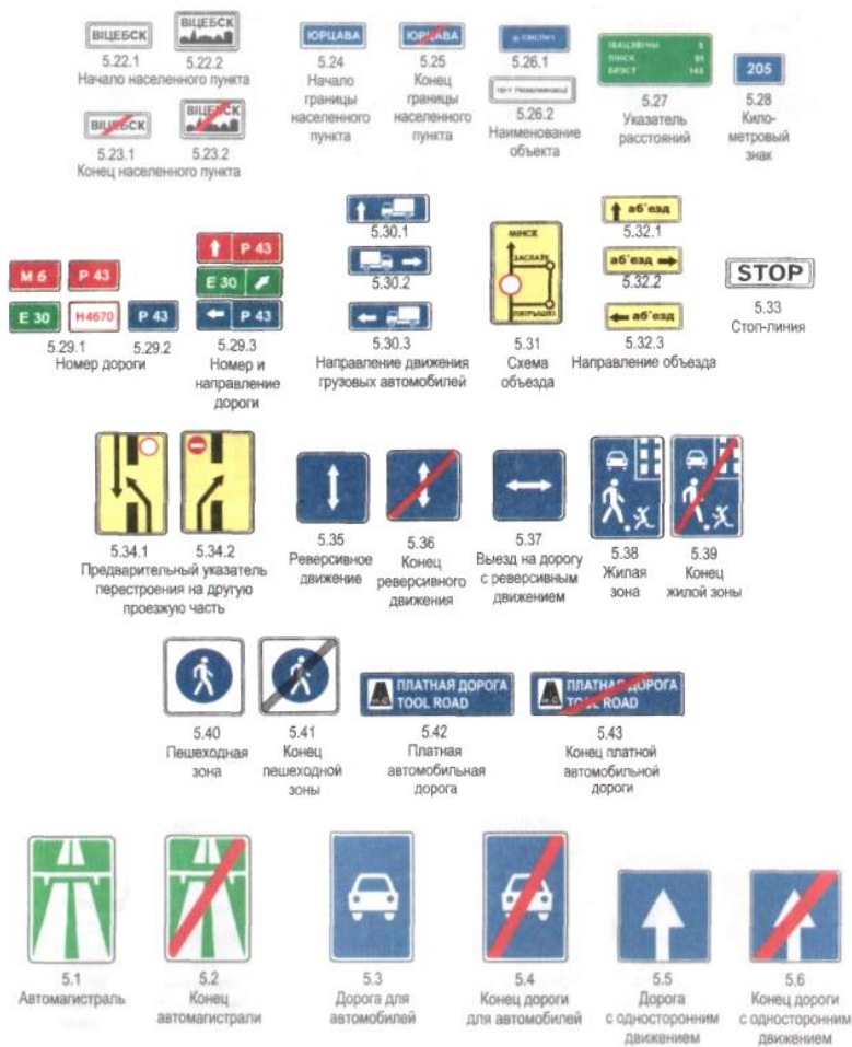
Рис. 1.45. Информационно-указательные знаки
