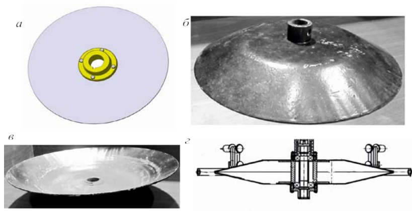
Рис.1. Типы распределяющих устройств: а – однодисковый; б – трапецидальный; в – тарельчатый; з – питатель с подвесками
