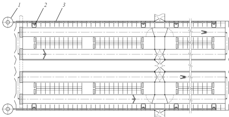
Рис. 4.17. Особенности планировки коровника беспривязно-буксового содержания при использовании комбинированного способа скармливания кормов:
