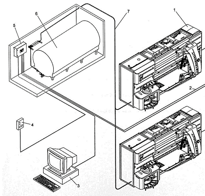
Рис. 6.4. Основные составляющие системы доения Astronaut: 1 – доильный робот; 2 – информационная сеть T4C; 3 – персональный компьютер; 4 – сигнализатор; 5 – контроллер CRS+; 6 – танк-охладитель молока; 7 – молокопровод
