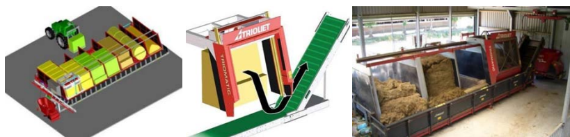
Рис. 4.9. Элементы роботизированной системы кормления КРС Triomatic
