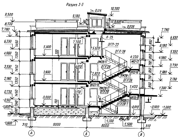
Рис. 6.12. Конструктивный разрез жилого дома по лестничной клетке
