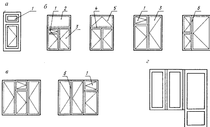
Рис. 5.3. Типы окон:
