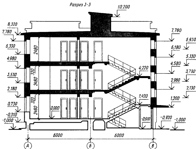
Рис. 6.11. Архитектурный разрез жилого дома по лестничной клетке
