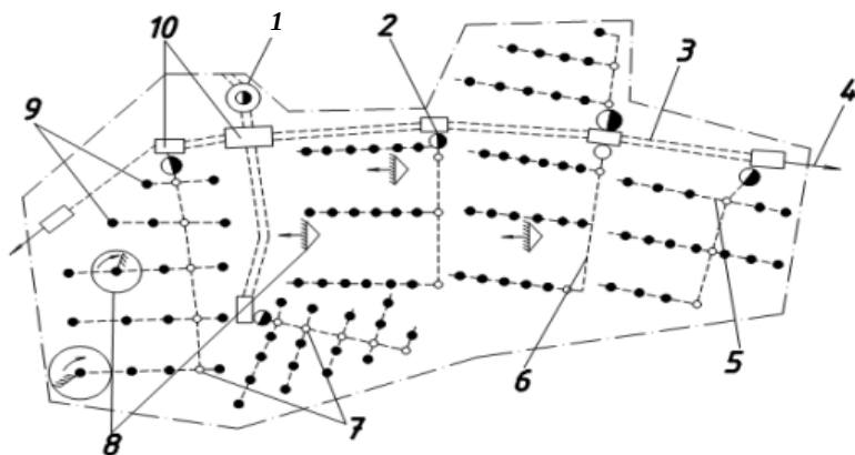
Рис. 9.2. Схема закрытой оросительной сети: 1 – головная насосная станция; 2 – насосная станция подкачки; 3, 5, 6 – магистральный, распределительный и полевой трубопроводы; 4 – концевые сбросы; 7 – колодцы с задвижками; 8 – дождевальные машины; 9 – гидранты; 10 – регулирующие бассейны
