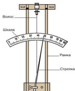
Рис. 1.2. Волосной гигрометр
