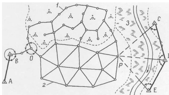
Рис. 4. Возможная схема привязки и развития съемочного обоснования площадного объекта: a – непосредственным примыканием точки O к опорным пунктам; б – прямой угловой засечкой точки P ; 1 – сеть теодолитных ходов в закрытой кустарником местности; 2 – триангуляционная сеть в открытой местности; 3 – заболоченная часть поймы реки; \Delta – исходные пункты
