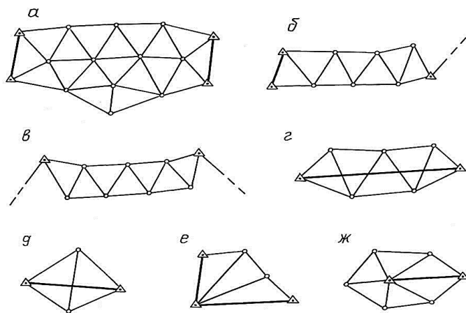
Рис. 1. Развитие съёмочной геодезической сети триангуляционными построениями: а – сеть треугольников между двумя исходными сторонами; б – цепочка треугольников между стороной и пунктом; в, г – цепочки треугольников между двумя пунктами; д – геодезический четырехугольник; е – вставка в угол; ж – центральная схема
